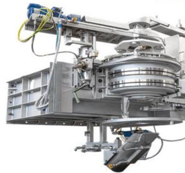
E-servo feeder
